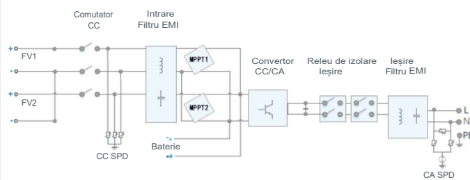
Schema circuitului
