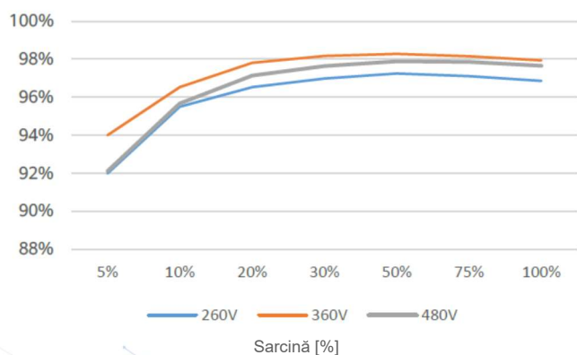
Curba eficienței
